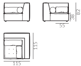
moduł narożny
